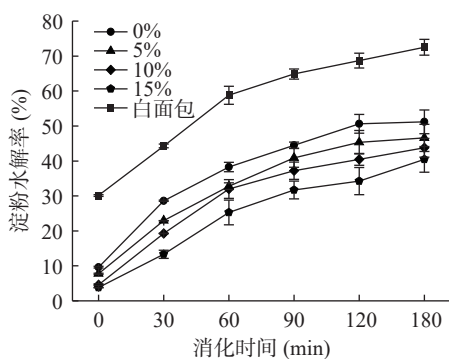
图6 黑米酒糟馒头的淀粉水解
