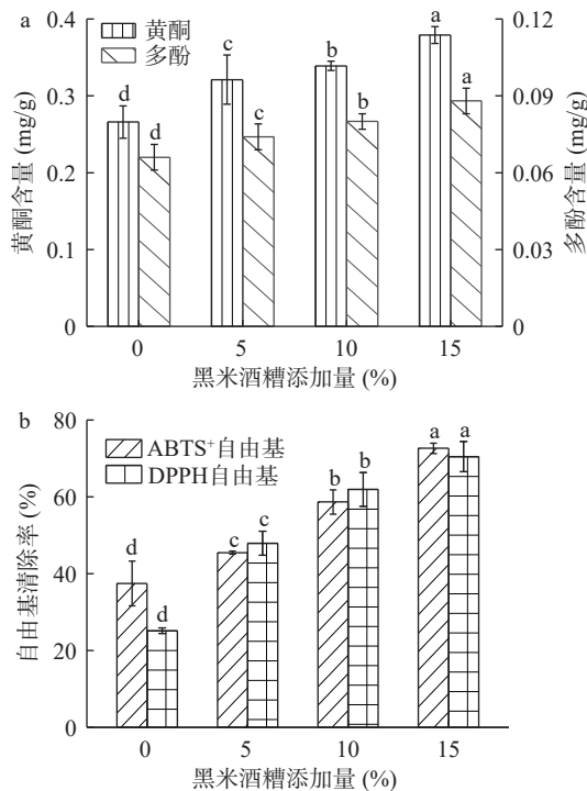
图 5 黑米酒糟馒头的抗氧化活性
