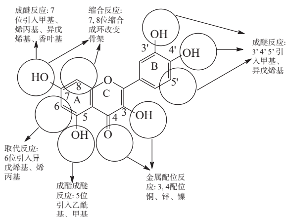
图 1 槲皮素及结构修饰 Fig.1 Quercetin and structural modification
