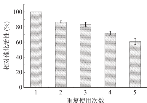
图 6 ZIF-67 的操作稳定性 Fig.6 Operational stability of ZIF-67
